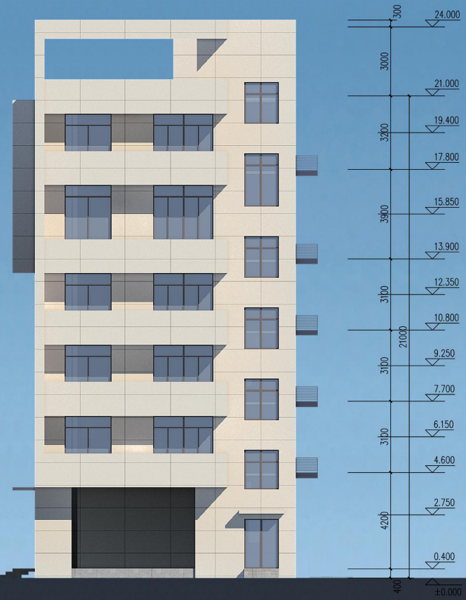
北立面
