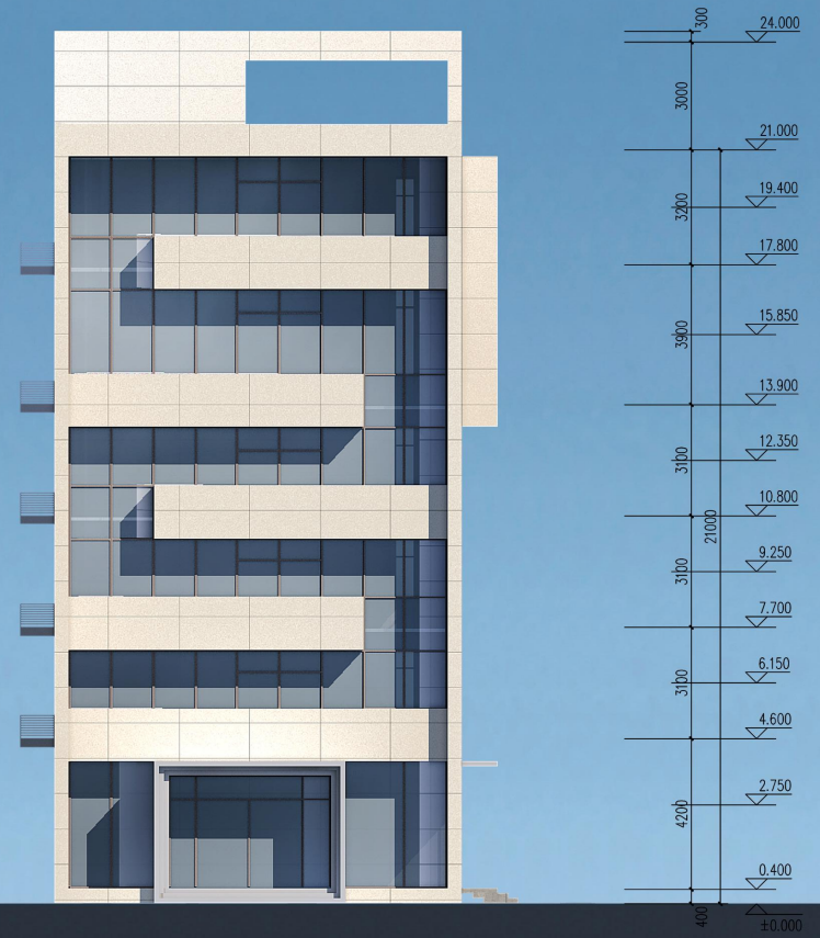
南立面
