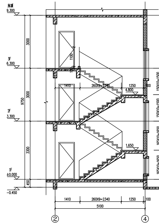
2-2剖面图 1:100
