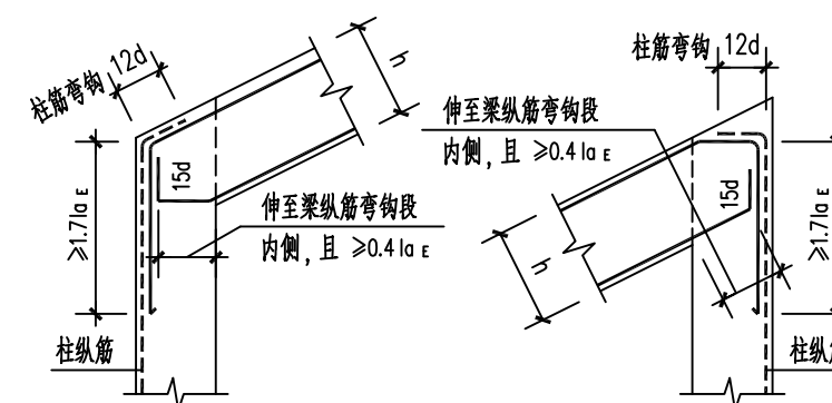
屋面框架斜梁的边支座纵筋锚固构造
