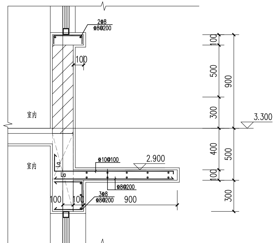
④ 雨披大样1 1:20
