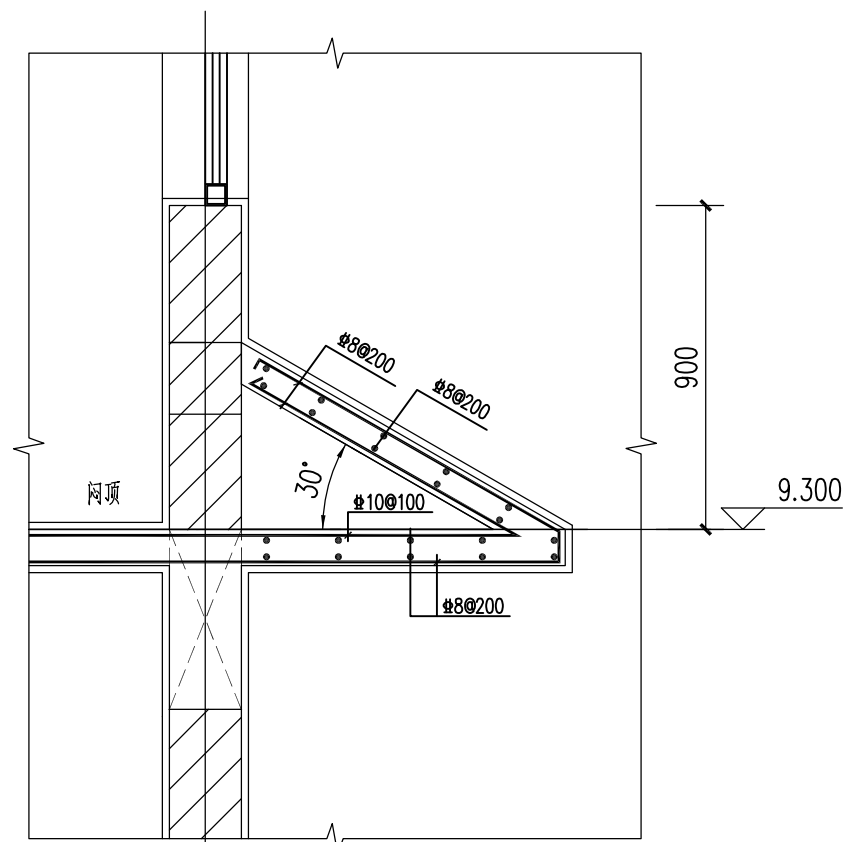
① 节点大样3 1:20
