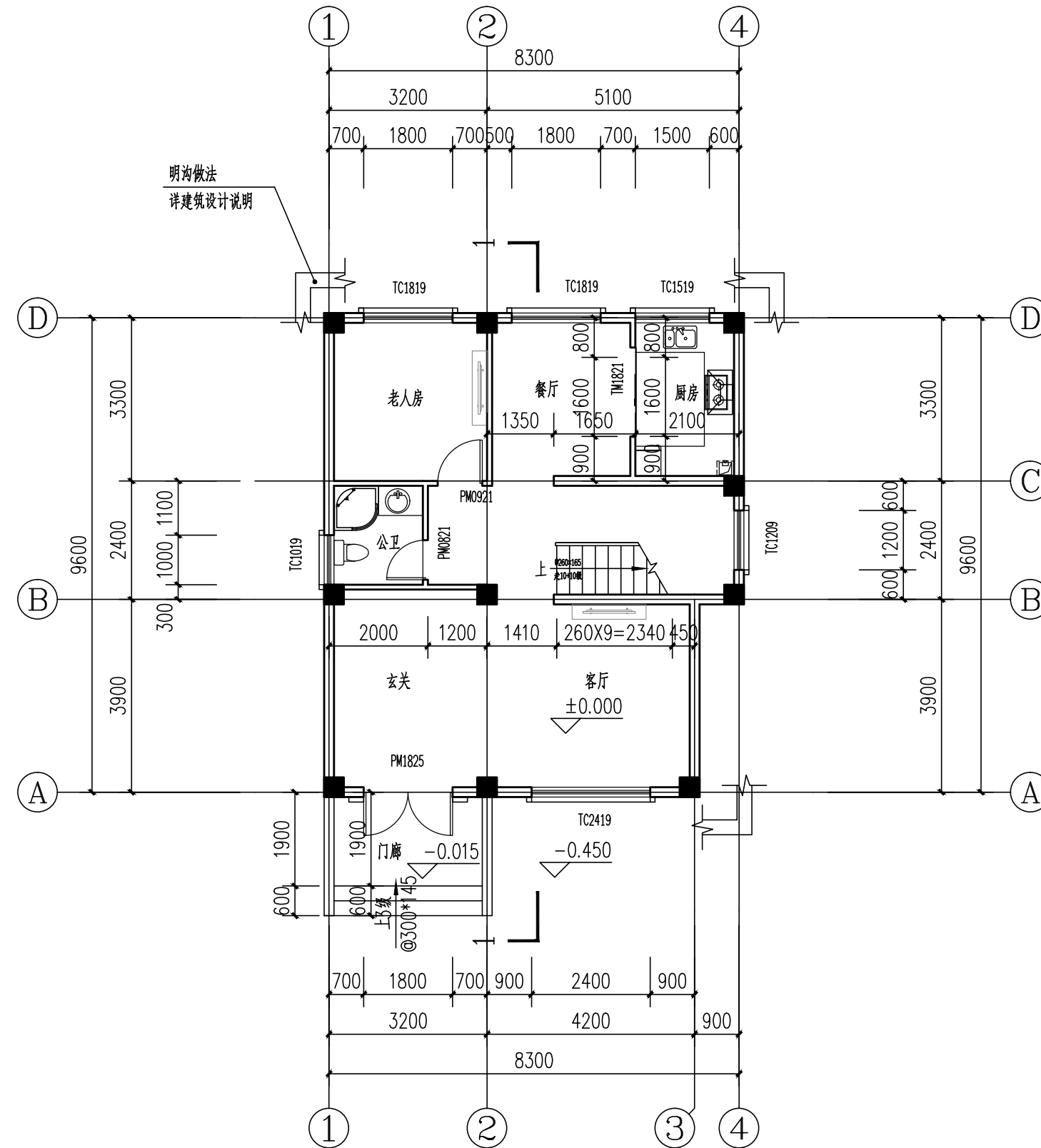
一层平面图 1:100
