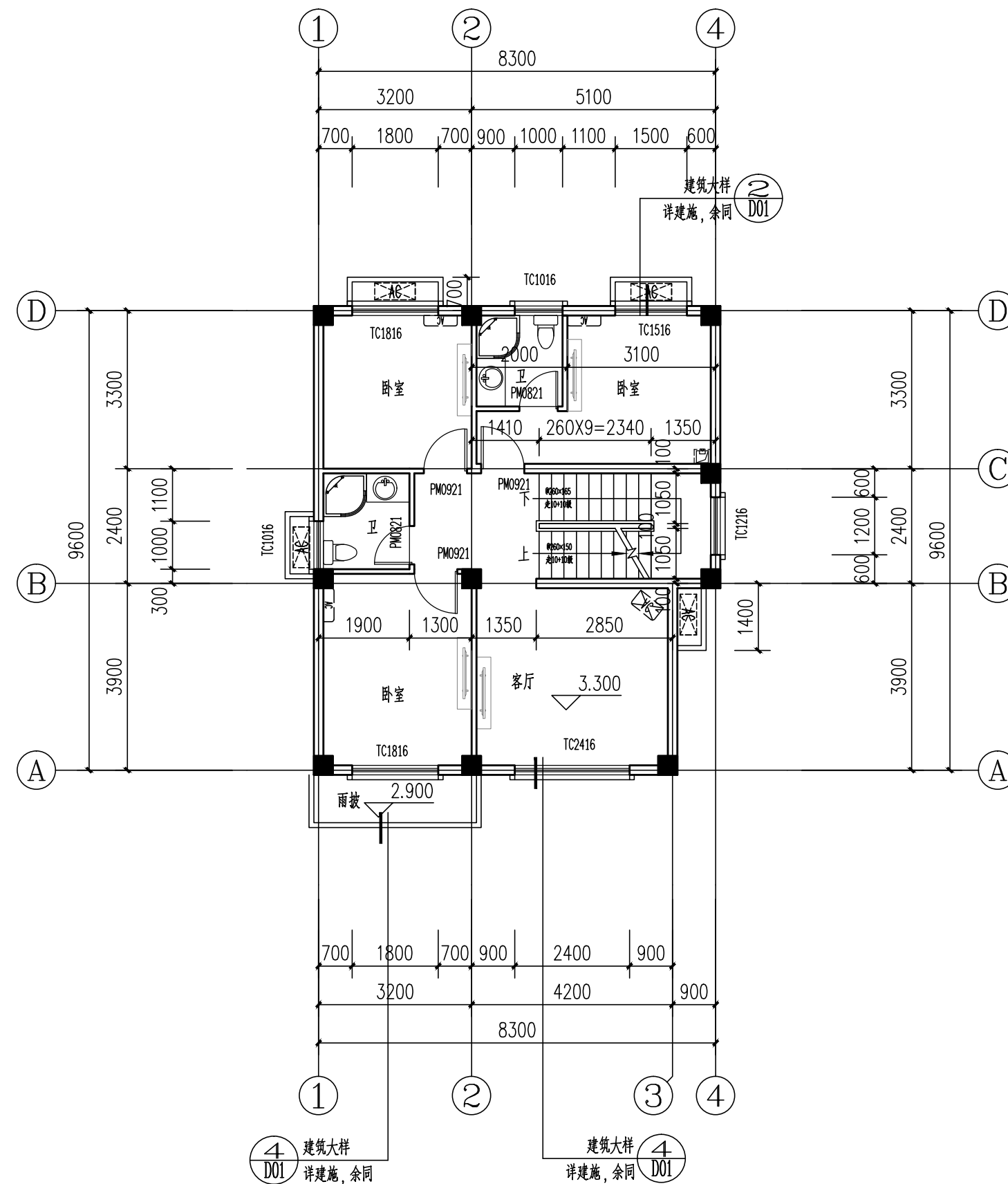
二层平面图 1:100
