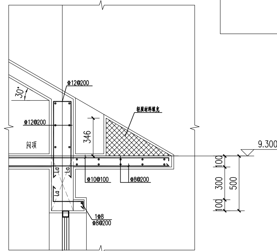
② 屋脊大样 1:20
