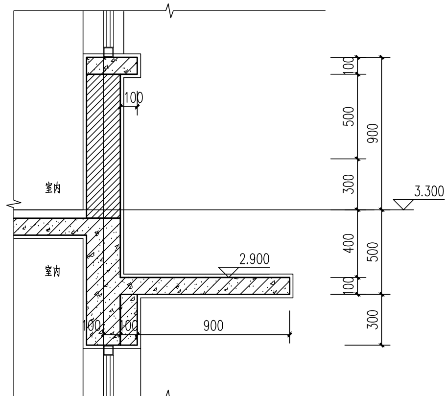
④ 雨披大样1 1:20
