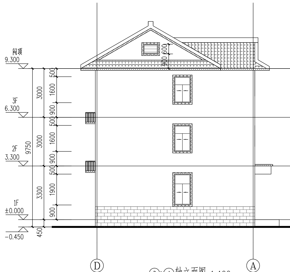
D~A轴立面图 1:100
