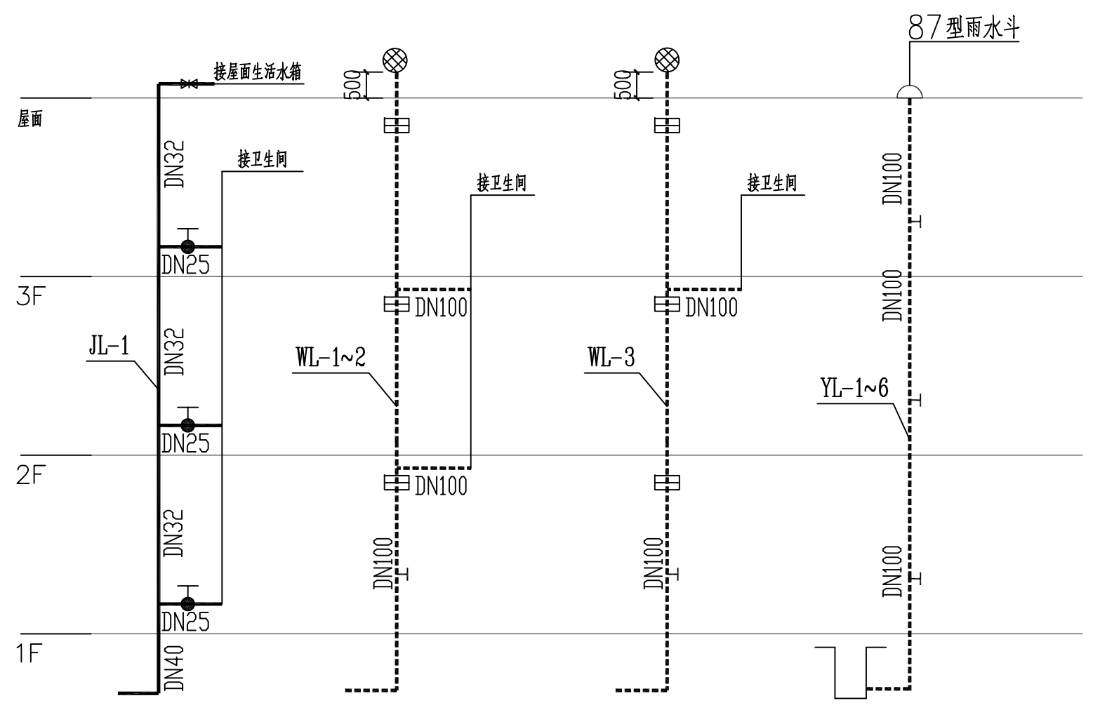
给排水系统图
