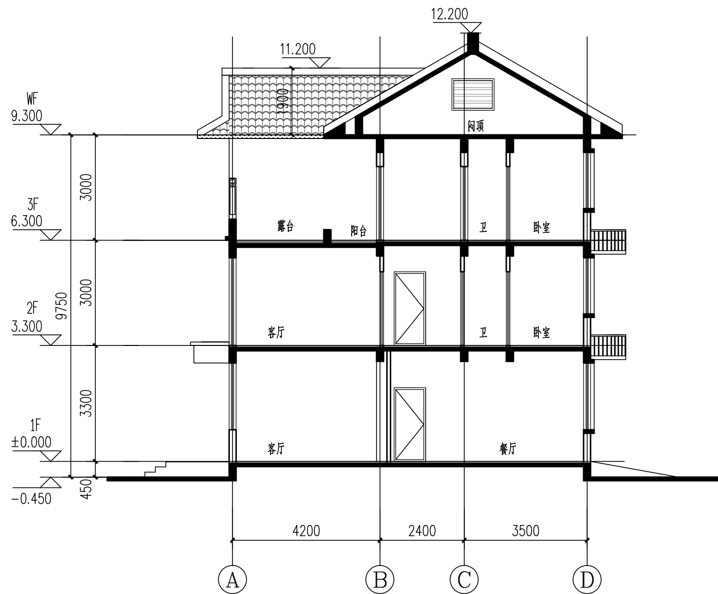
1-1剖面图 1:100
