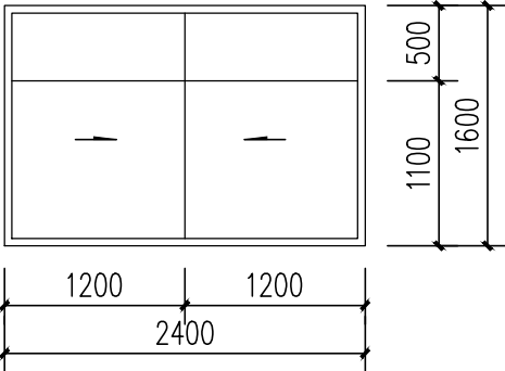
TC2416 1:50
