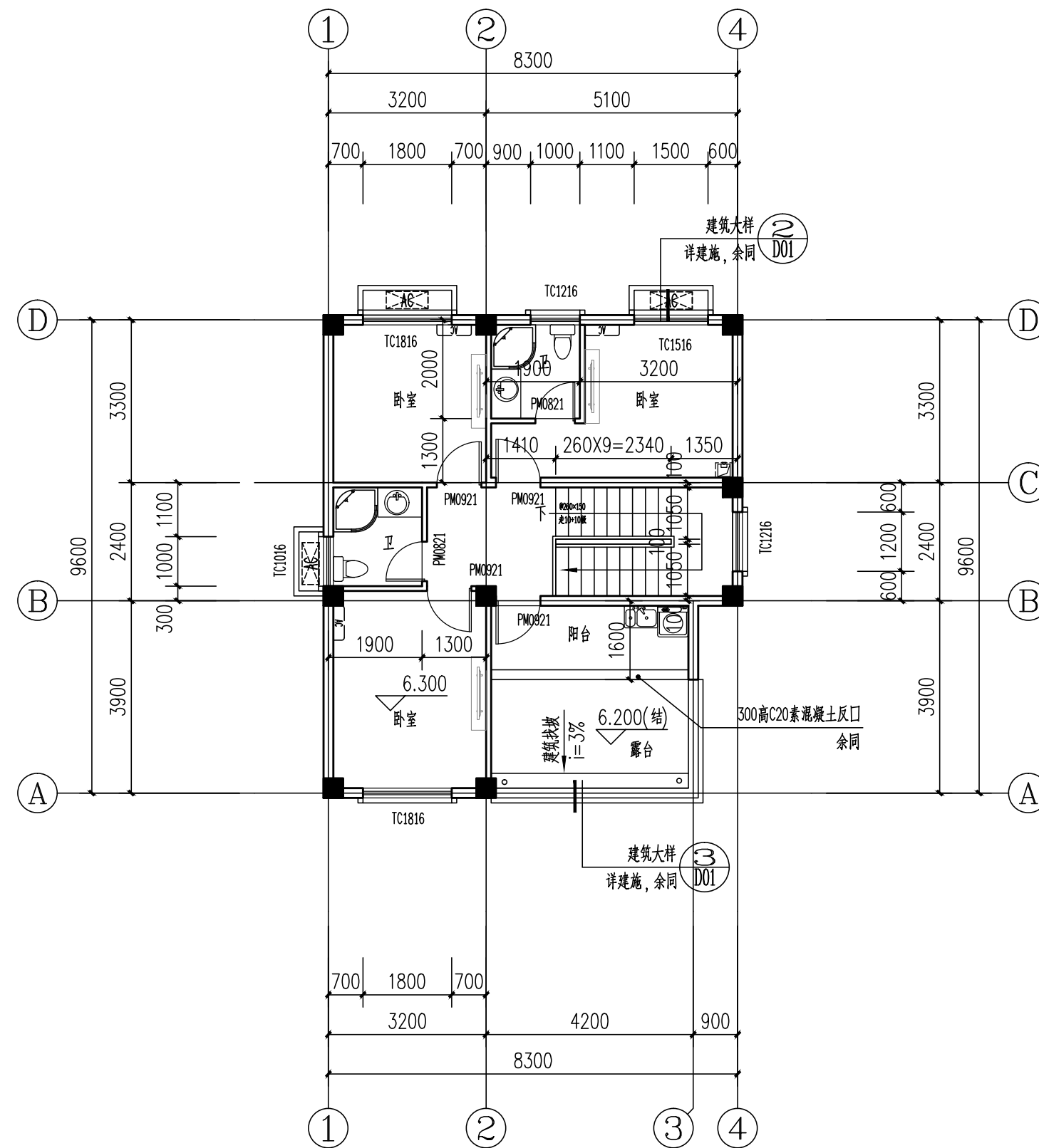
三层平面图 1:100
