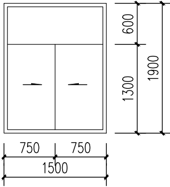
TC1519 1:50
