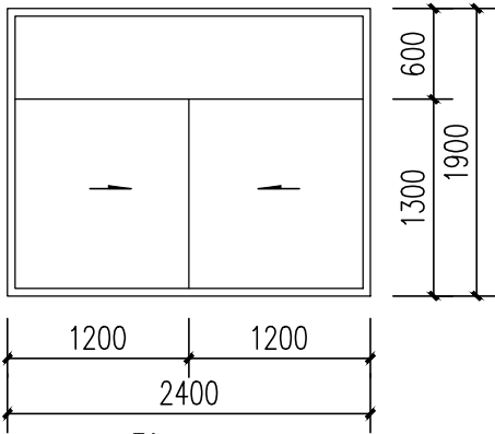
TC2419 1:50
