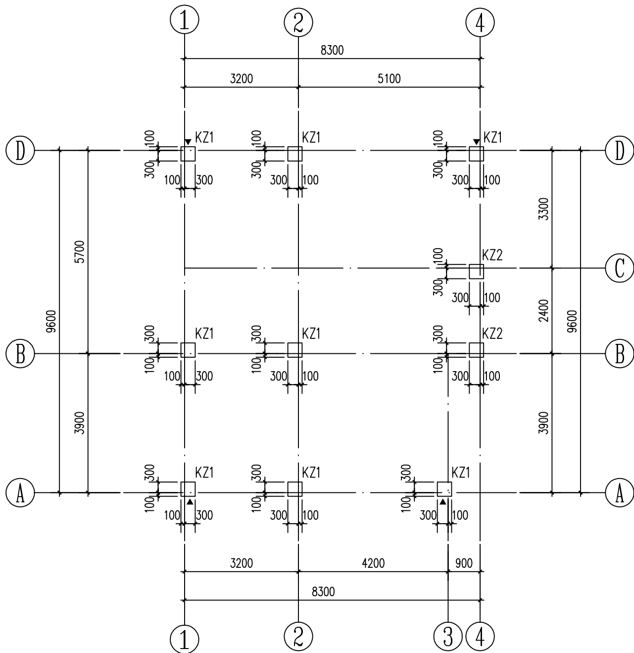
一~二层柱平面布置图 1:100
