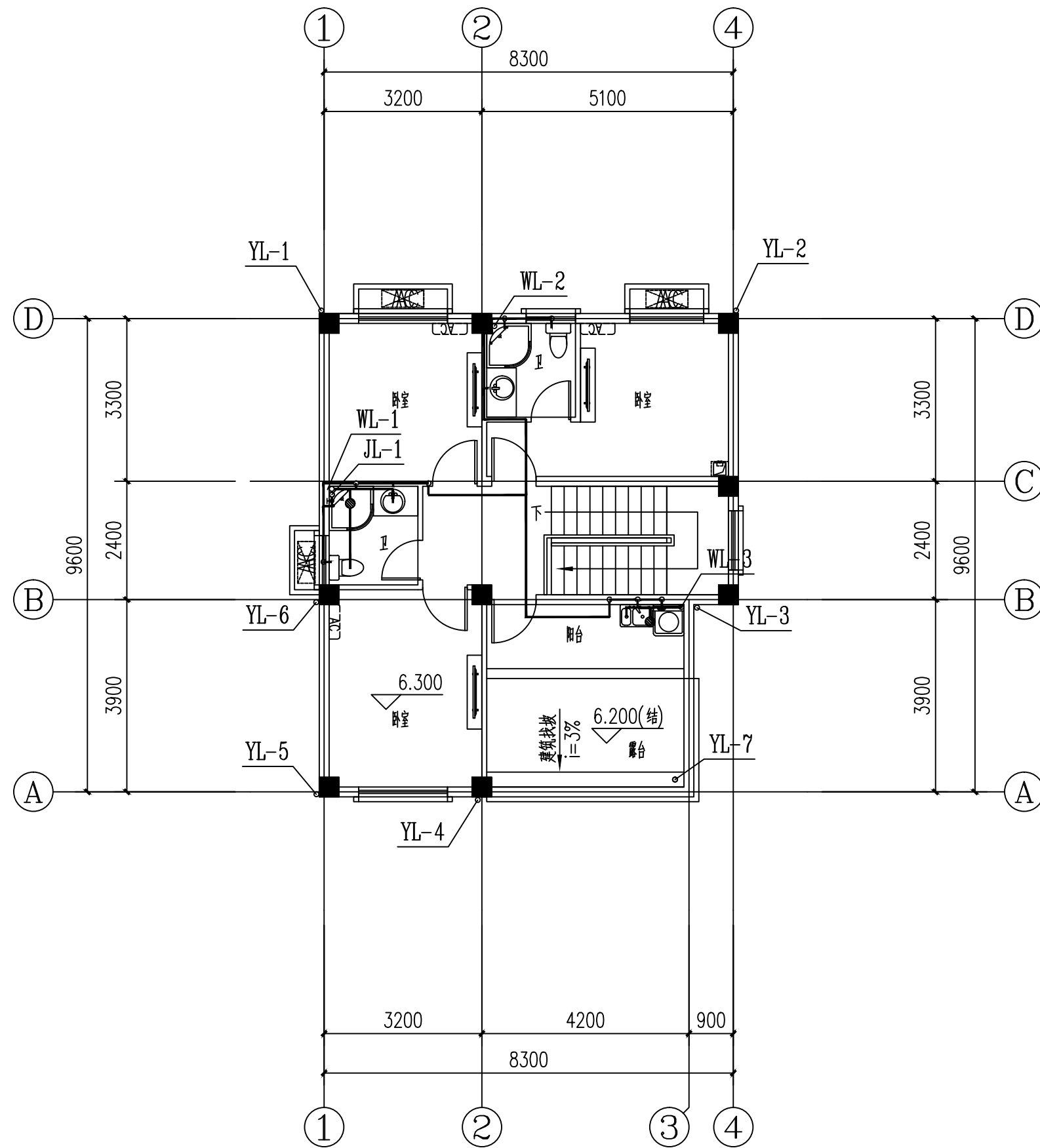
三层给排水平面图 1:100
