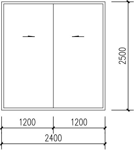
TM2425 1:50
