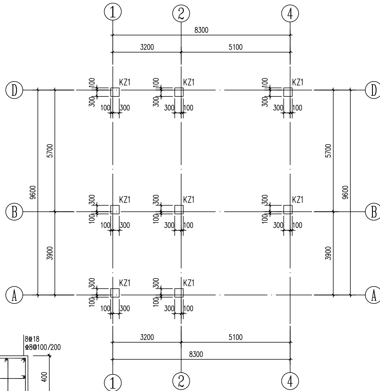
三层柱平面布置图 1:100
